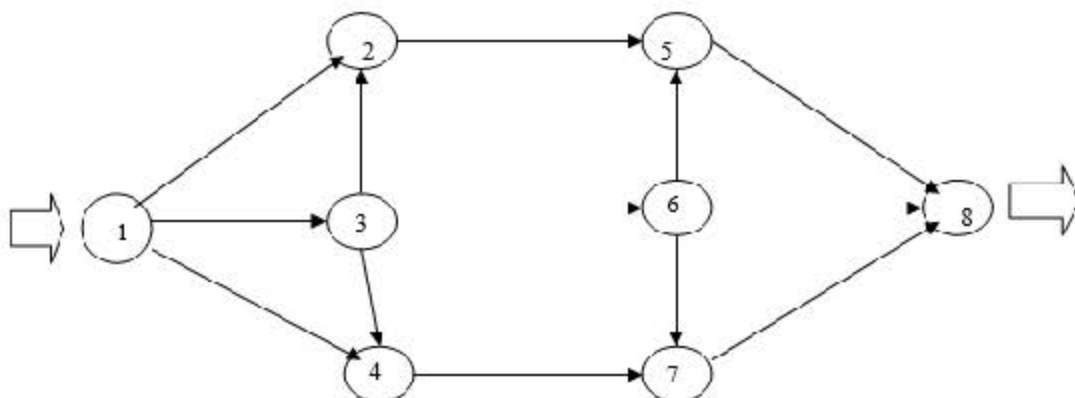
Рис. 3.11. Транспортная сеть к задаче о максимальном потоке
