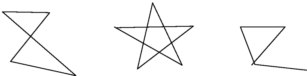
Рис. 3.6. Примеры графов
