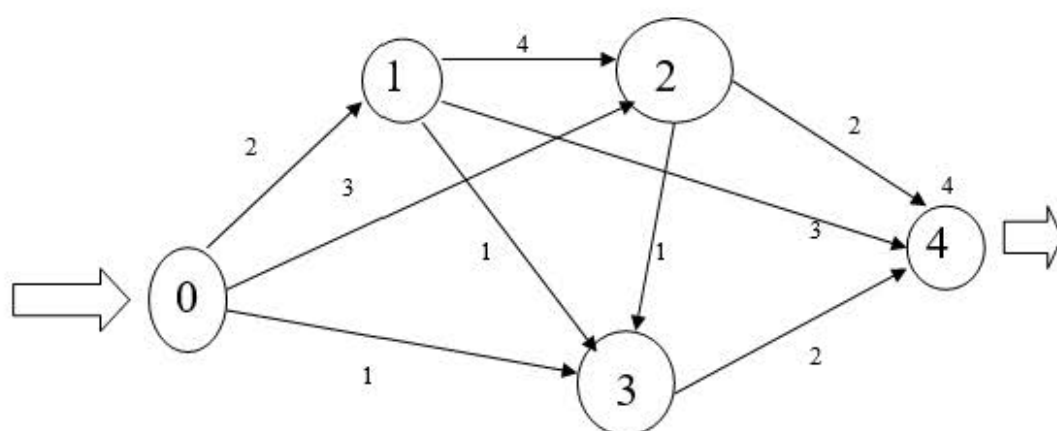
Рис. 3.9. Исходные данные к задаче о максимальном потоке
