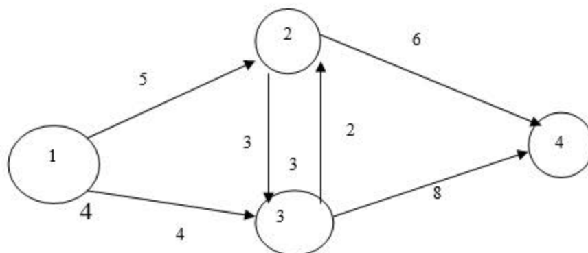
Рис. 3.10. Исходные данные к задаче о кратчайшем пути
